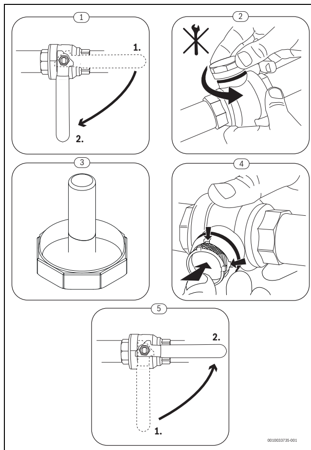
Bild 44 Siebreinigung
