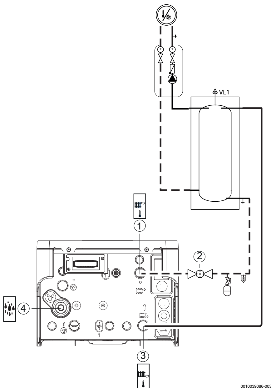
Bild 20 Anschluss der Inneneinheit an die Heizungsanlage
