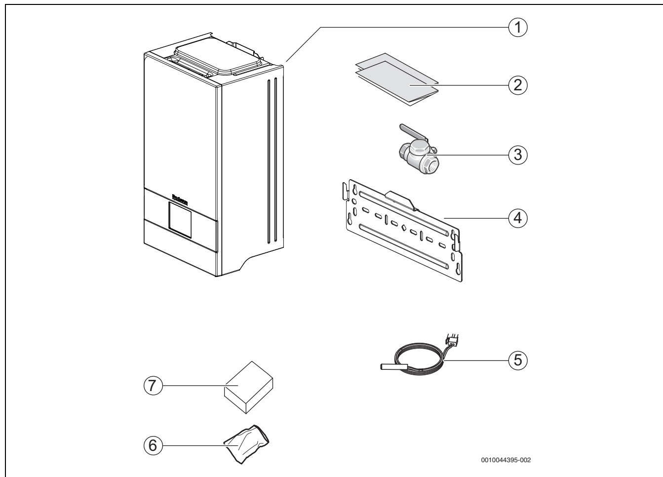
Bild 1 Lieferumfang
