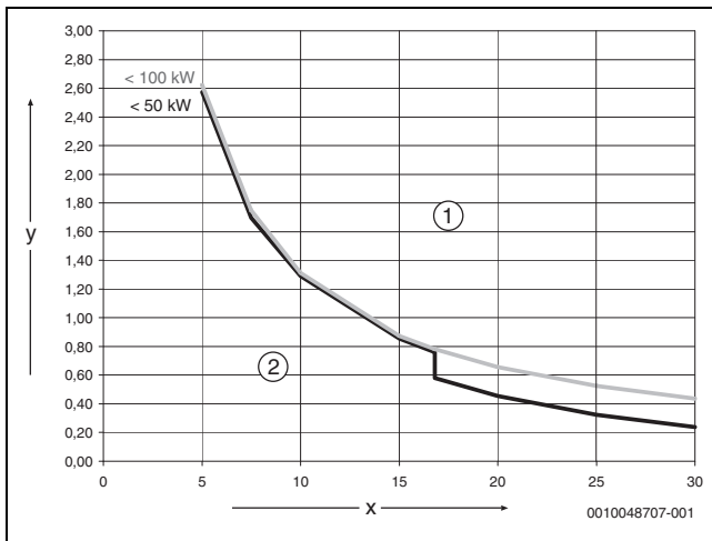
Bild 8 Wärmepumpen < 50 kW < 100 kW
