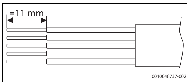
Bild 28 Abisolieren der Adern für den Netzanschluss
