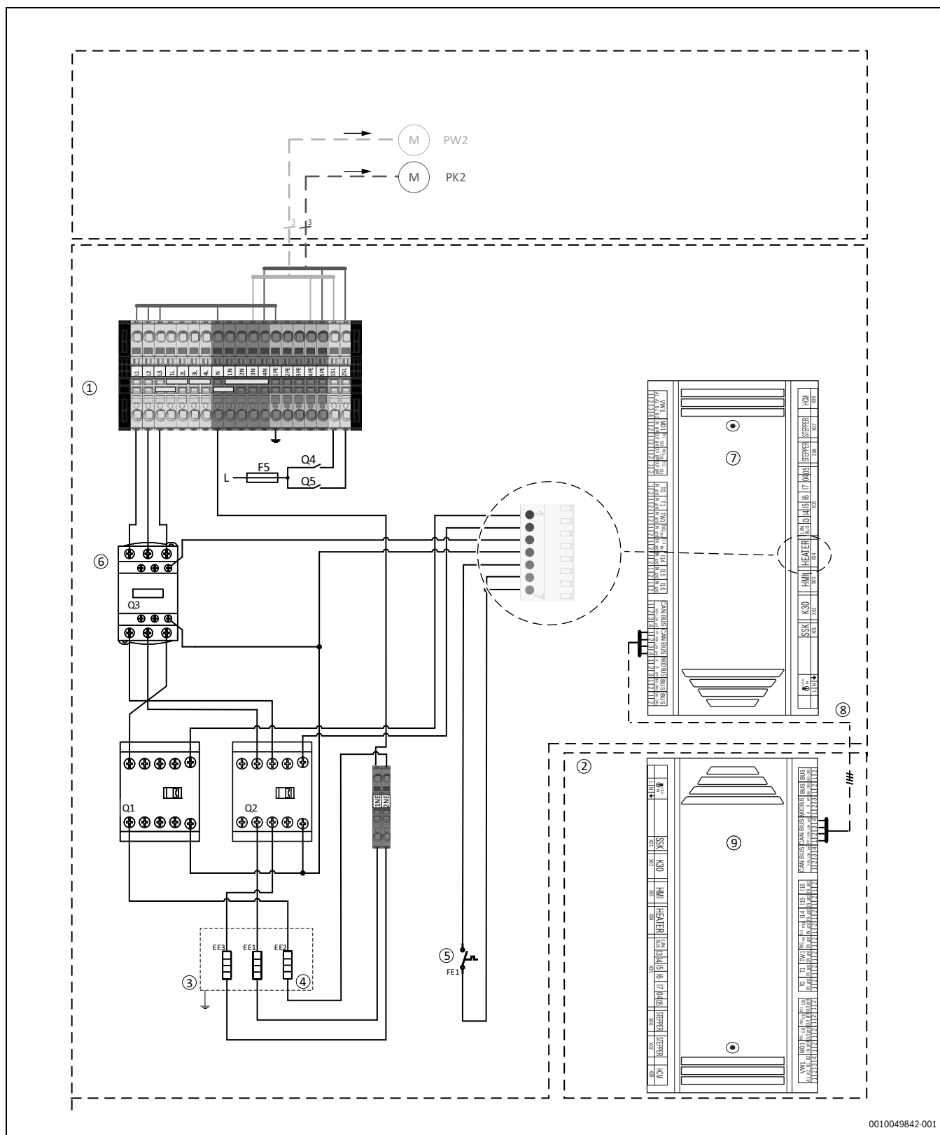
Bild 50 Spannungsversorgung Inneneinheit
