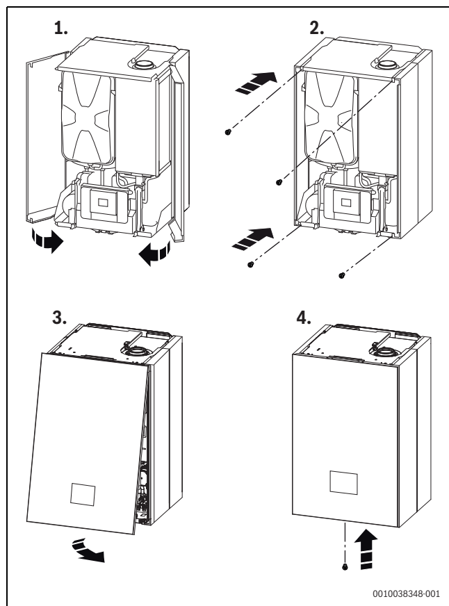
Bild 47 Verkleidung montieren
