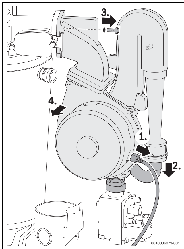
Bild 59 Gebläse mit Mischeinrichtung ausbauen
