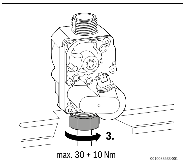
Bild 83 Anzugsdrehmoment beachten
