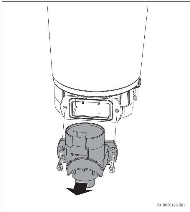
Bild 68 Prüfföffnung öffnen
