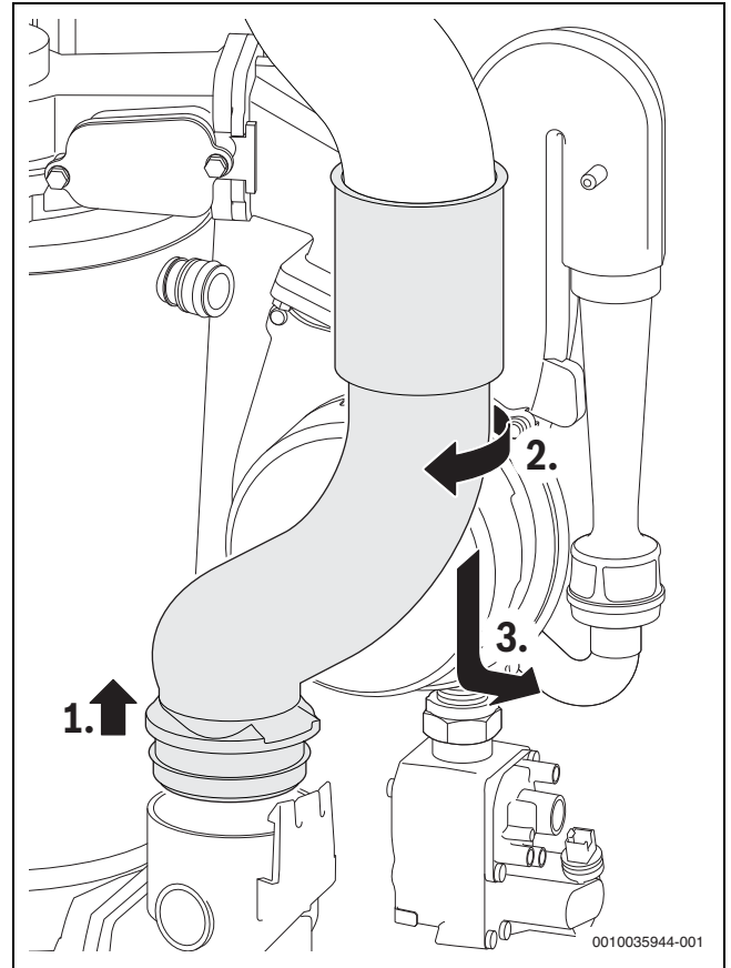
Bild 58 Abgasrohr ausbauen
