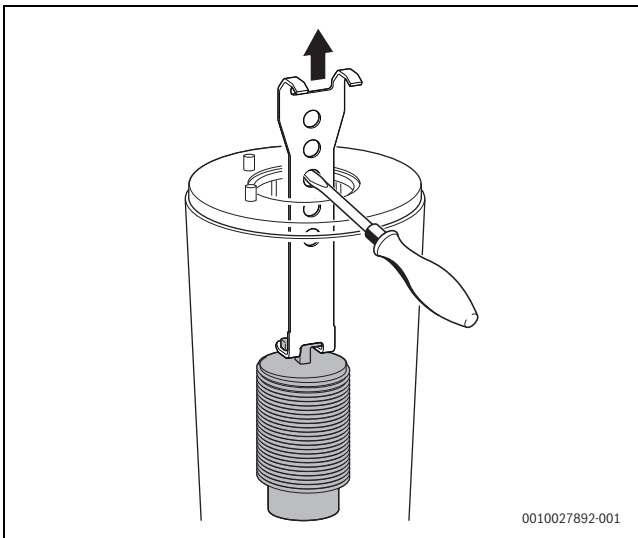
Bild 64 Unteren Verdrängungskörper herausnehmen
