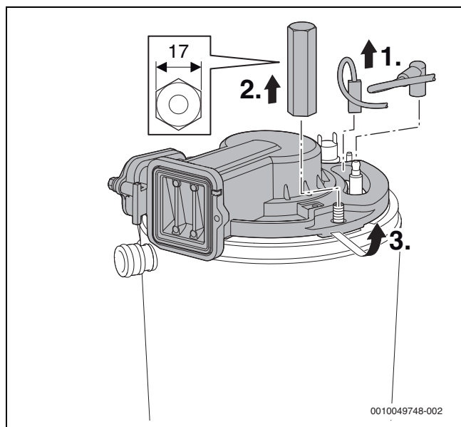
Bild 60 Brennerdeckel lösen
