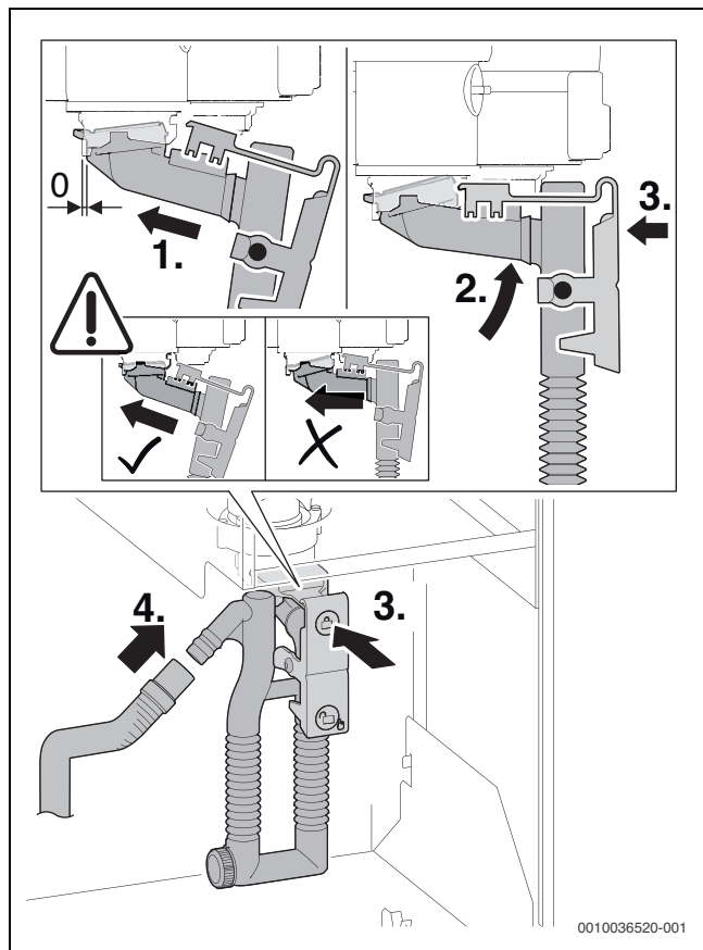
Bild 75 Kondensatsiphon einsetzen
