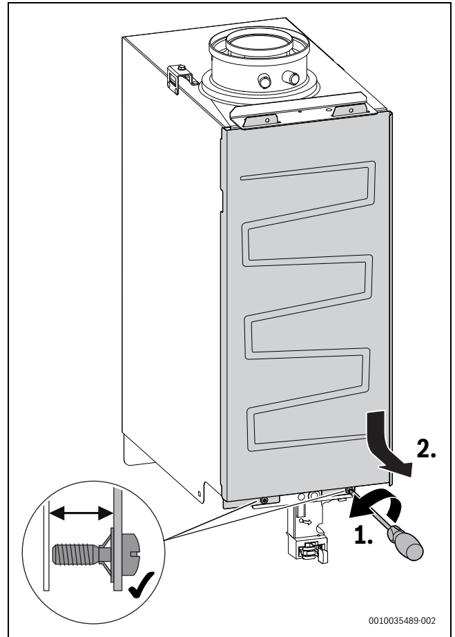
Bild 51 Brennerhaube abnehmen
