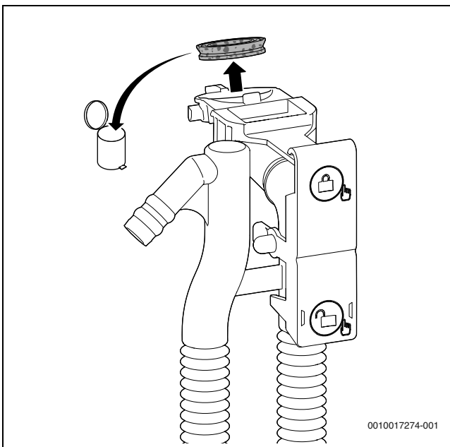
Bild 72 Dichtung oben am Kondensatsiphon entfernen
