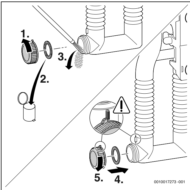
Bild 71 Kondensatsiphon reinigen
