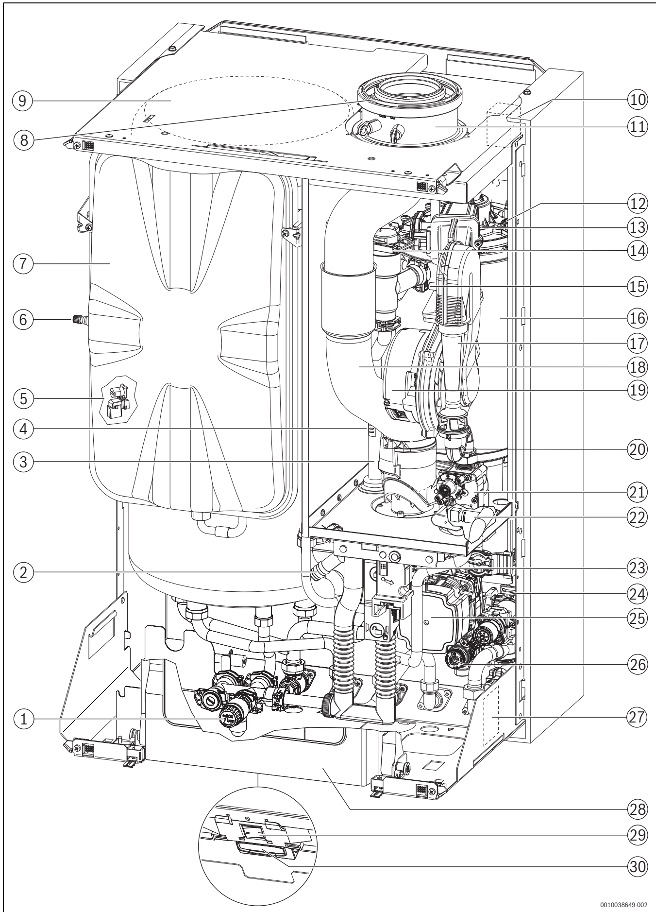
Bild 4 Produktübersicht
