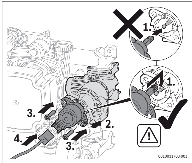
Bild 89 Motor am 3-Wege-Ventil einbauen (Variante mit Schrauben)
