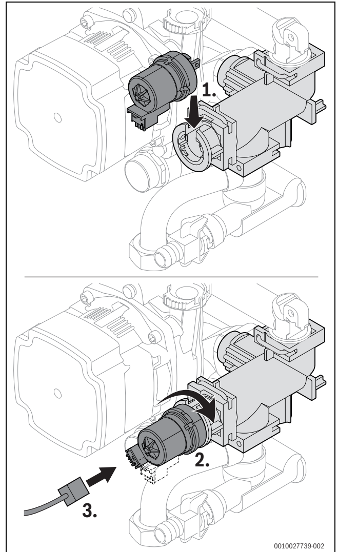
Bild 87 Motor am 3-Wege-Ventil einbauen (Variante ohne Schrauben)
