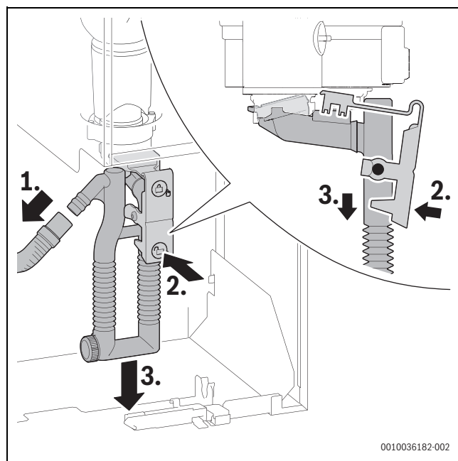
Bild 70 Kondensatsiphon ausbauen
