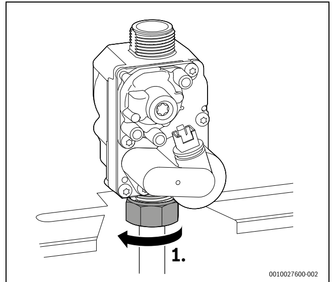
Bild 80 Überwurfmutter lösen
