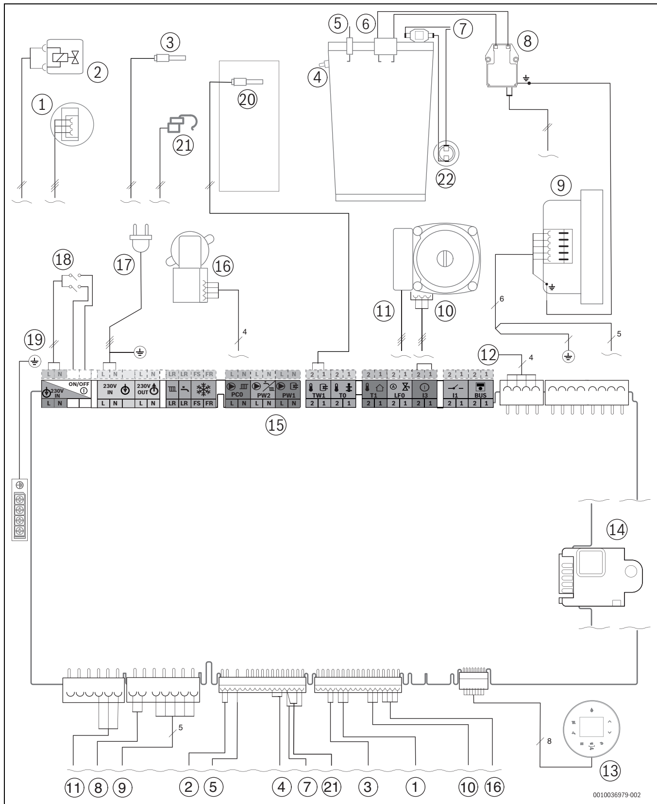
Bild 92 Elektrische Verdrahtung
