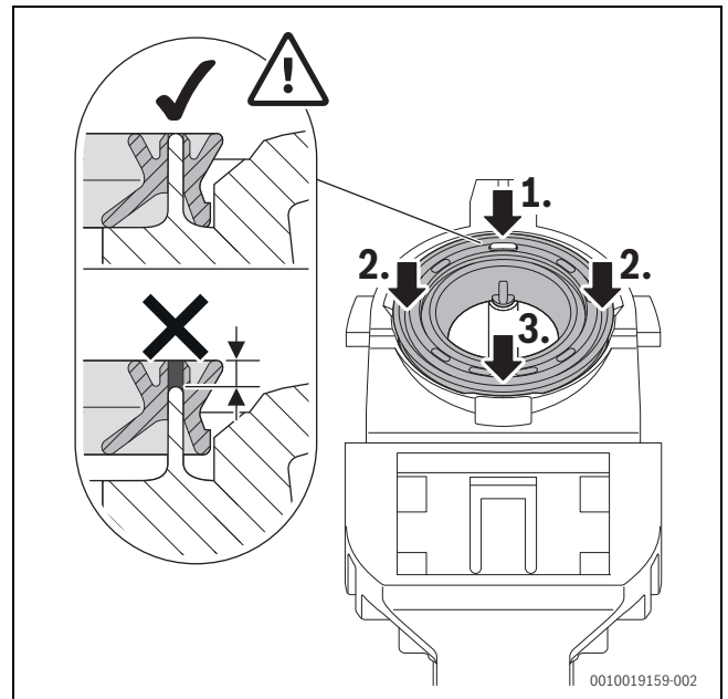
Bild 74 Dichtung andrücken
