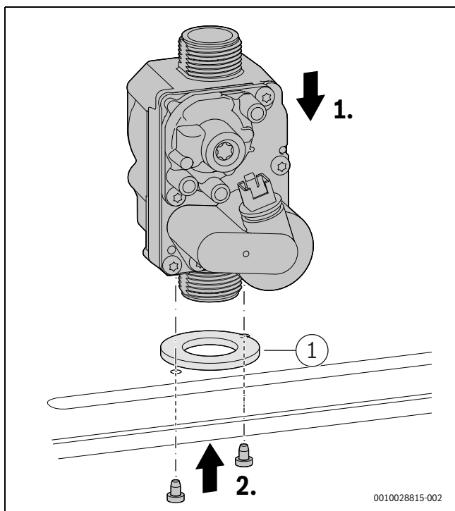
Bild 82 Gasarmatur einbauen
